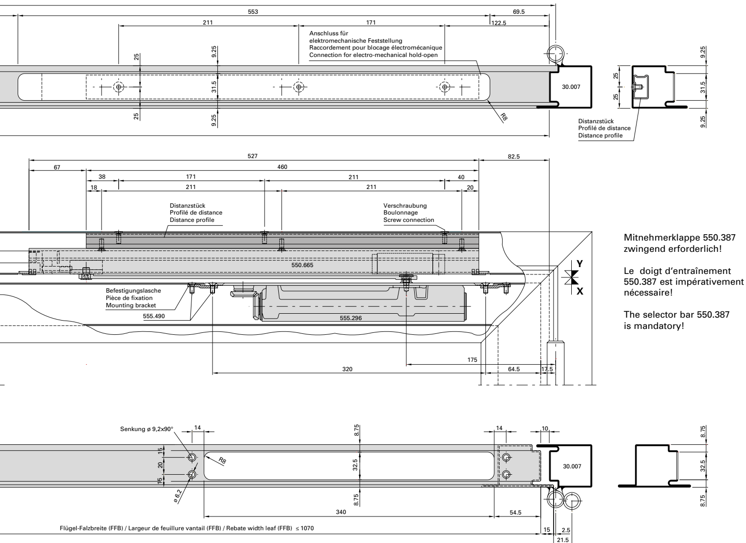
Abbildung: Gleitschiene 550.665
