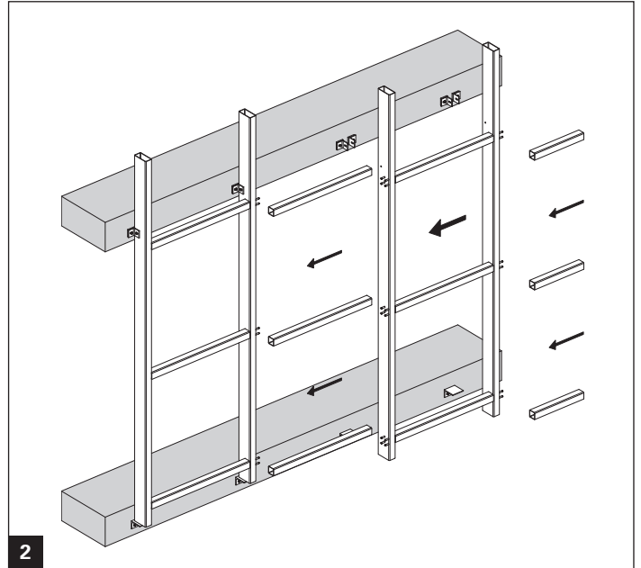
Rahmenbauweise / Steckbauweise Construction par éléments / construction modulaire Unitised construction / Push-on construction Costruzione a elementi / costruzione modulare
