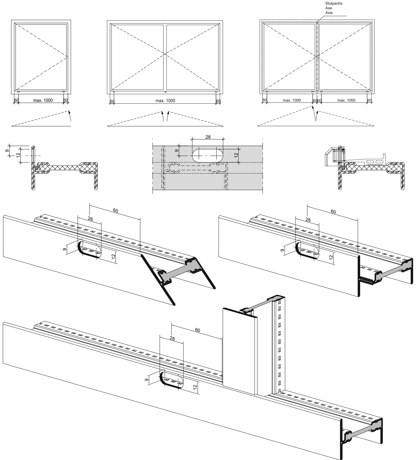
Einbau mit 499.469
