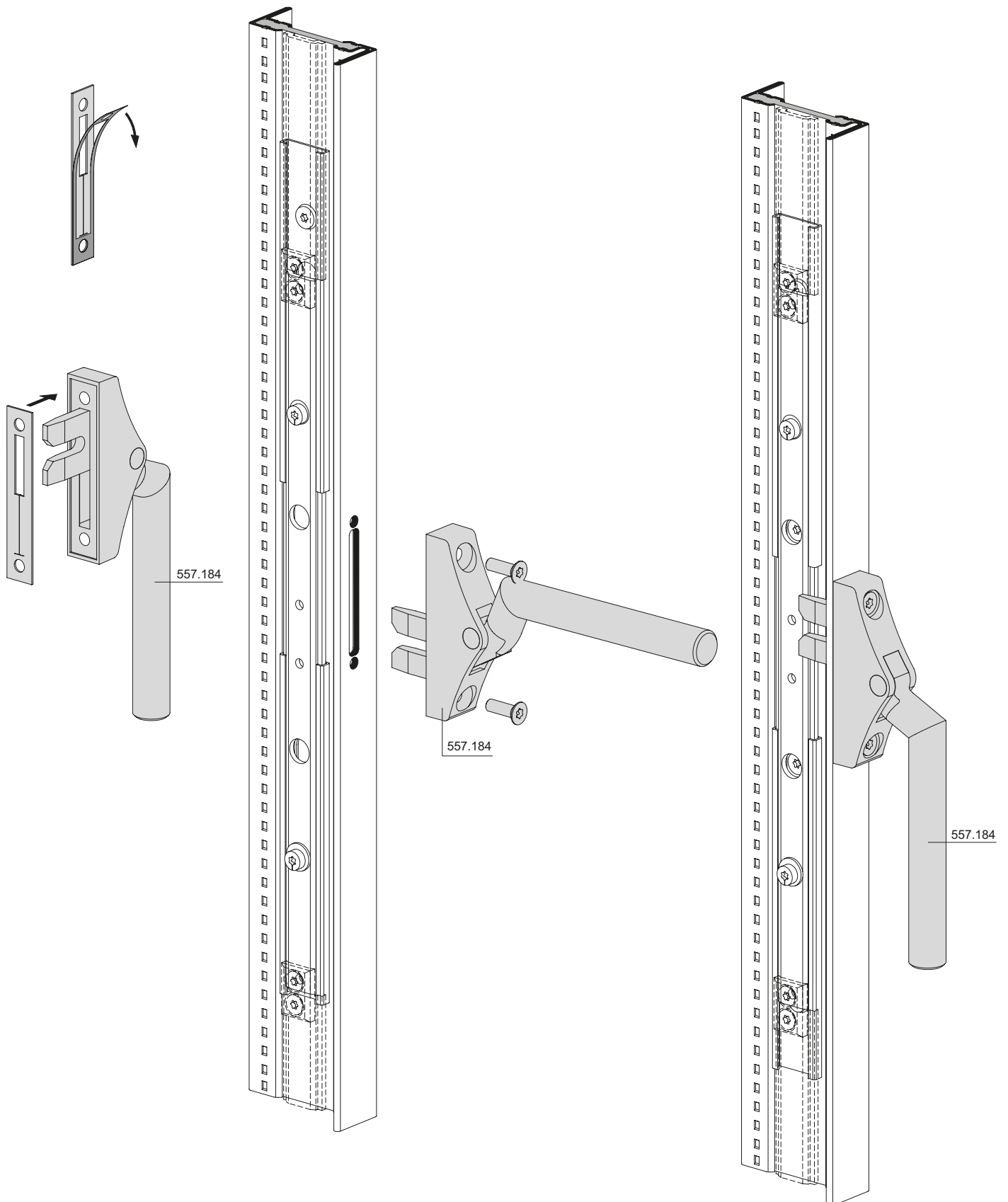
Einbau Fenstergriff 557.184 / 557.185 / 557.300
