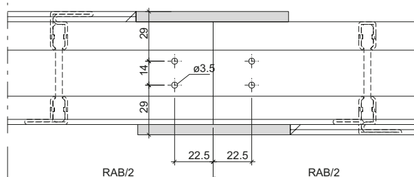
Flügel oben (Ansicht von oben) Vantail en haut (vue du haut) Sash at top (view from above)
