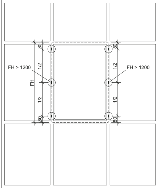
Ausführung mit Band
