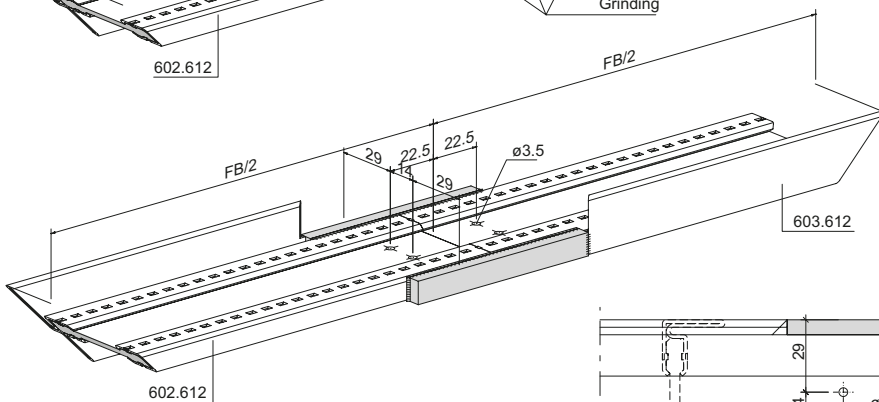
Flügel oben (Ansicht von oben) Vantail en haut (vue du haut) Sash at top (view from above)
