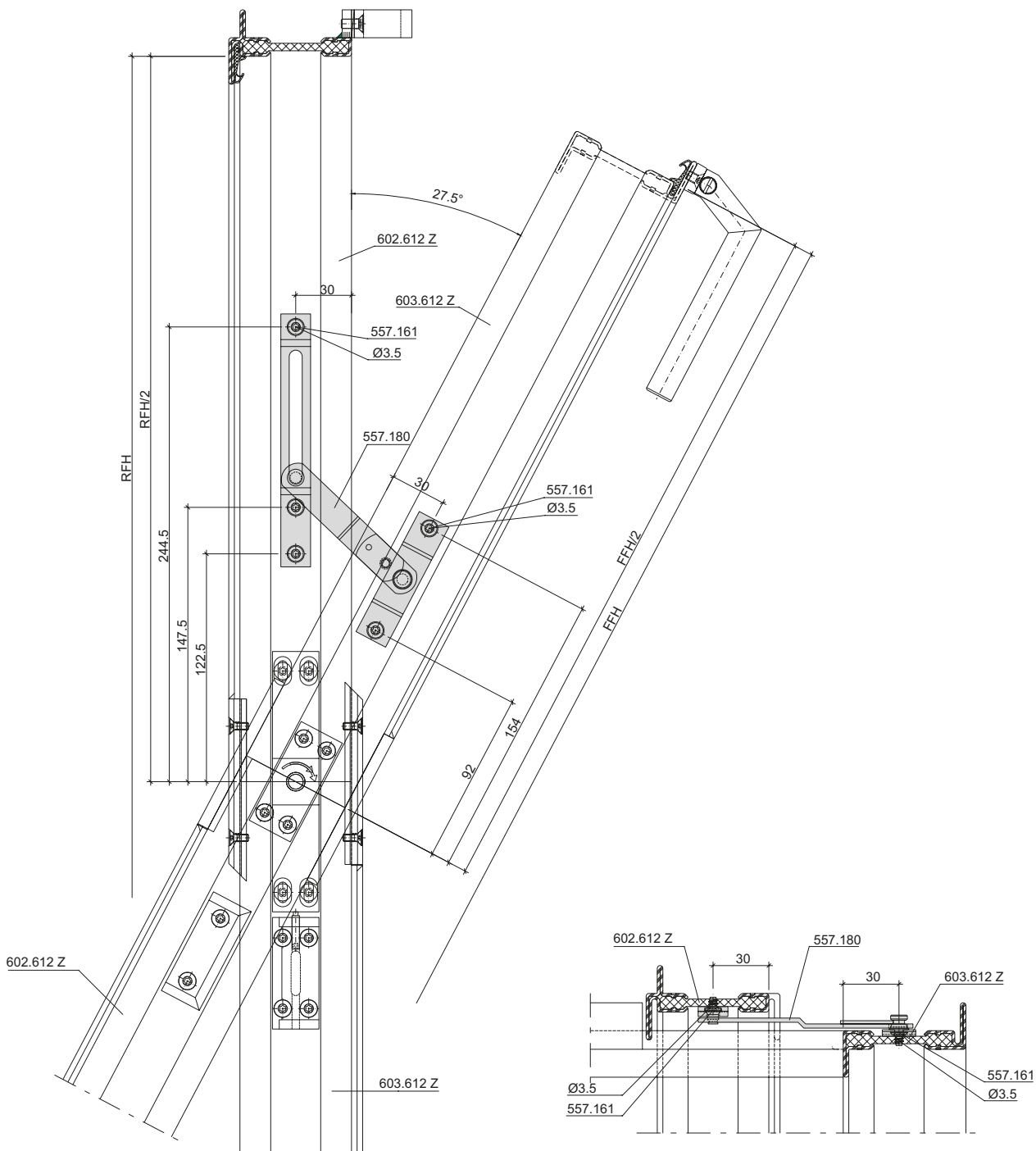
Angle d'ouverture 557.180 (en fonction de la position de montage)
