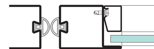
Kyvné dveře
