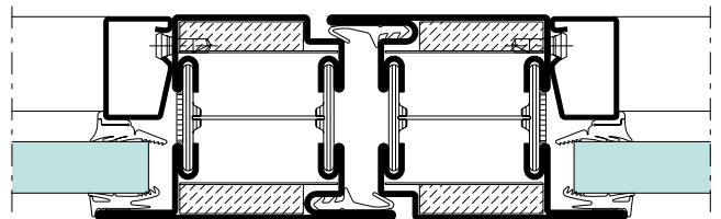
Janisol 2 EI30
