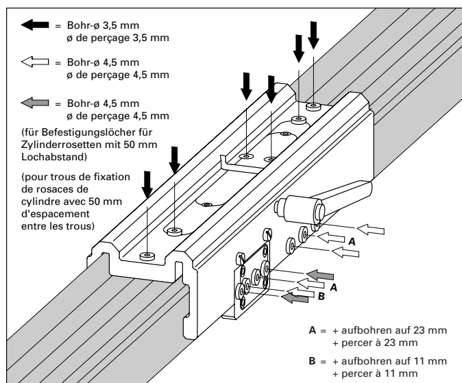
Abb. 2 Hauptschloss Fig. 2 Serrure principale
