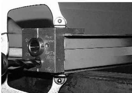
Abb. 23 Standflügel unten (Sockelprofil 601.685)
