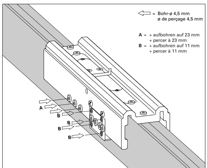
Abb. 3 Hauptschloss Fig. 3 Serrure principale
