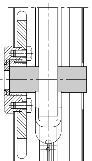
Abb. 38c Stulpschraube eindrehen Fig. 38c Poser la vis de la tête
