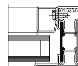
ŘEZ D
